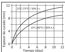
Diagrama 1: Velocidad de curado del Sikaflex - 256
