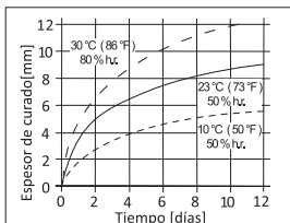
Diagrama 1: Velocidad de curado Sikaflex-260 N
